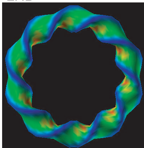
LHD
