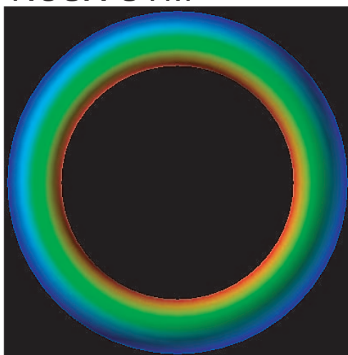
NCSX-SYM
