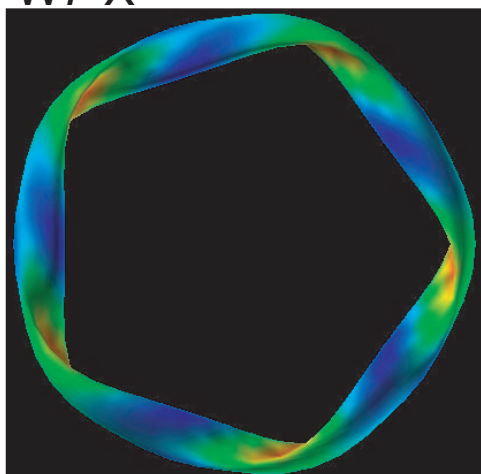
W7-X
