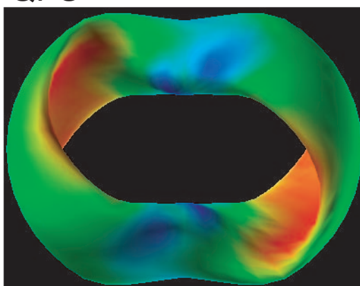
QPS
