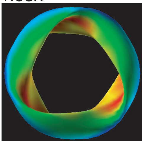
NCSX
